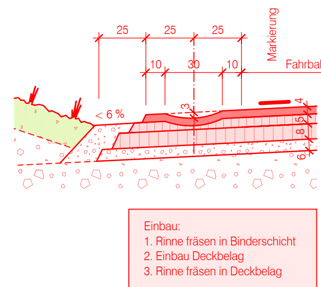
Detail 1 1:20 Belagsrinne
